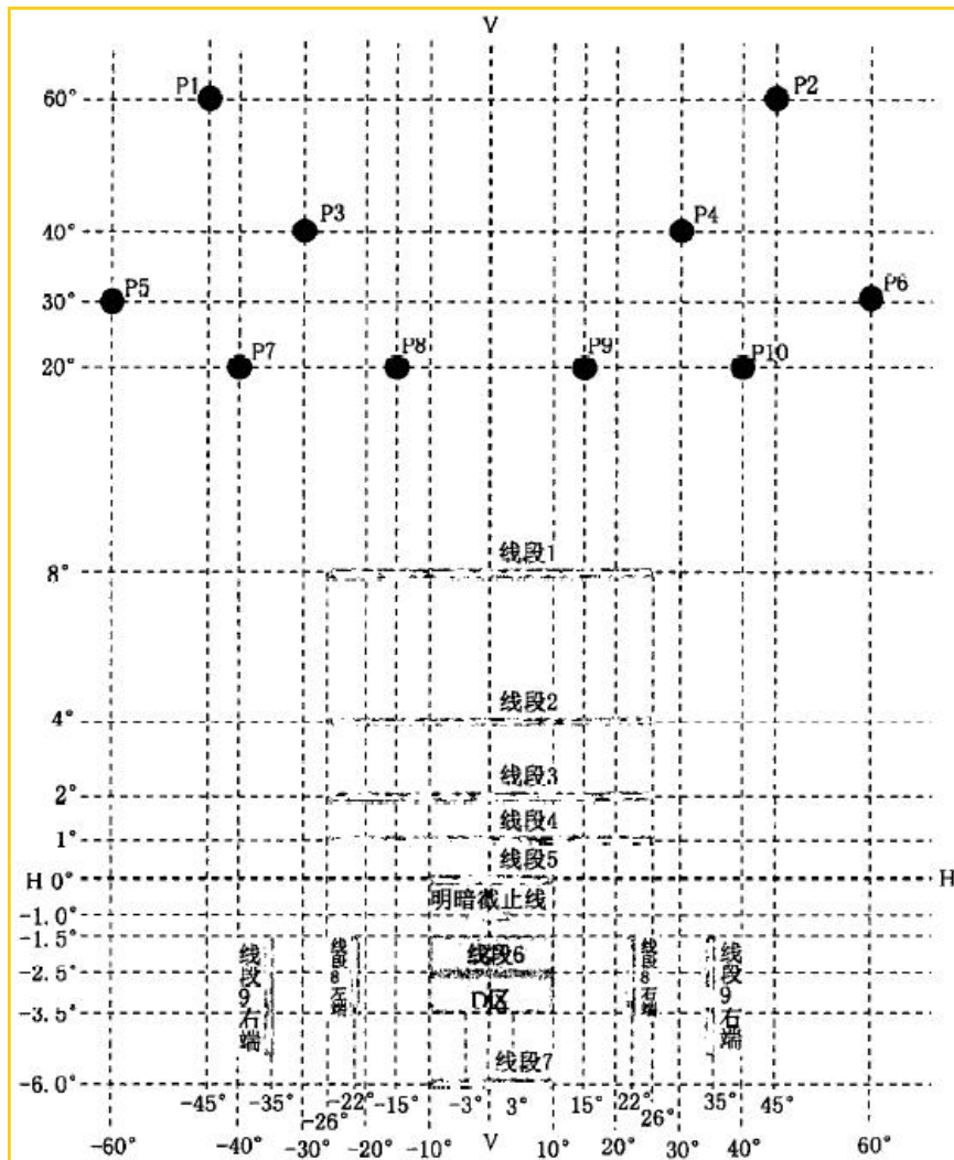
图 2 F3 级前雾灯配光屏幕
